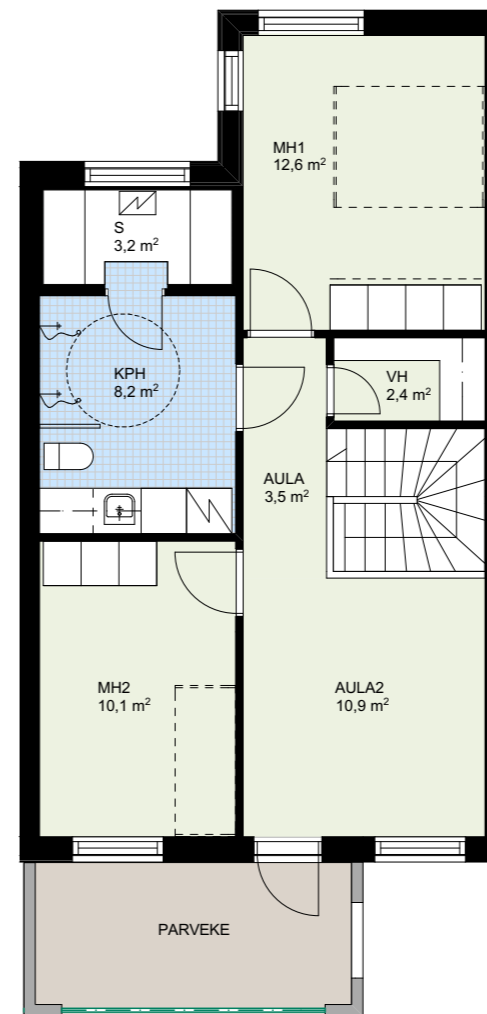
HSTO 2 2.krs 1:100
