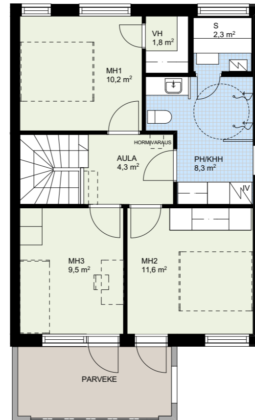
HSTO 4 2.krs 1:100
