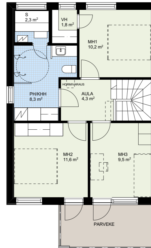
HSTO 1 2.krs 1:100
