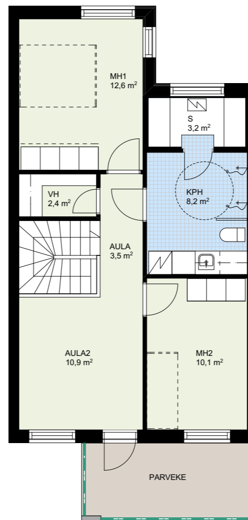
HSTO 3 2.krs 1:100
