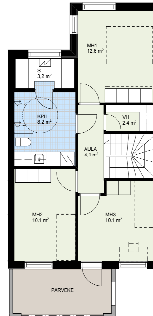
HSTO 2 2.krs 1:100
